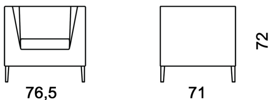
poltroncina armchair Kg 27 - mc 0,35
